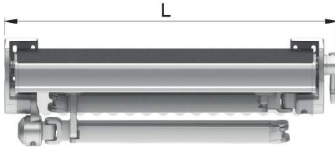
L para máquina por fuera con suplemento 80081660 L for gear outside with supplement 80081660 L pour treuil dehors avec supplément 80081660 L per arganella esteriore con supplemento 80081660
